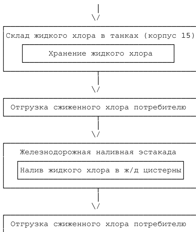
Рис. 18. Схема основных технологических потоков хлора на декларируемом объекте - основной производственной площадке Энского комбината по производству каустической соды
