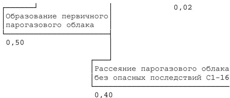
Рис. 11. Пример "Дерева событий" (фрагмент) при аварии на установке первичной переработки нефти - разрушении дегидрататора ДГ-1 (90 т нефти, T < 100 град. С, P < 1 МПа)
